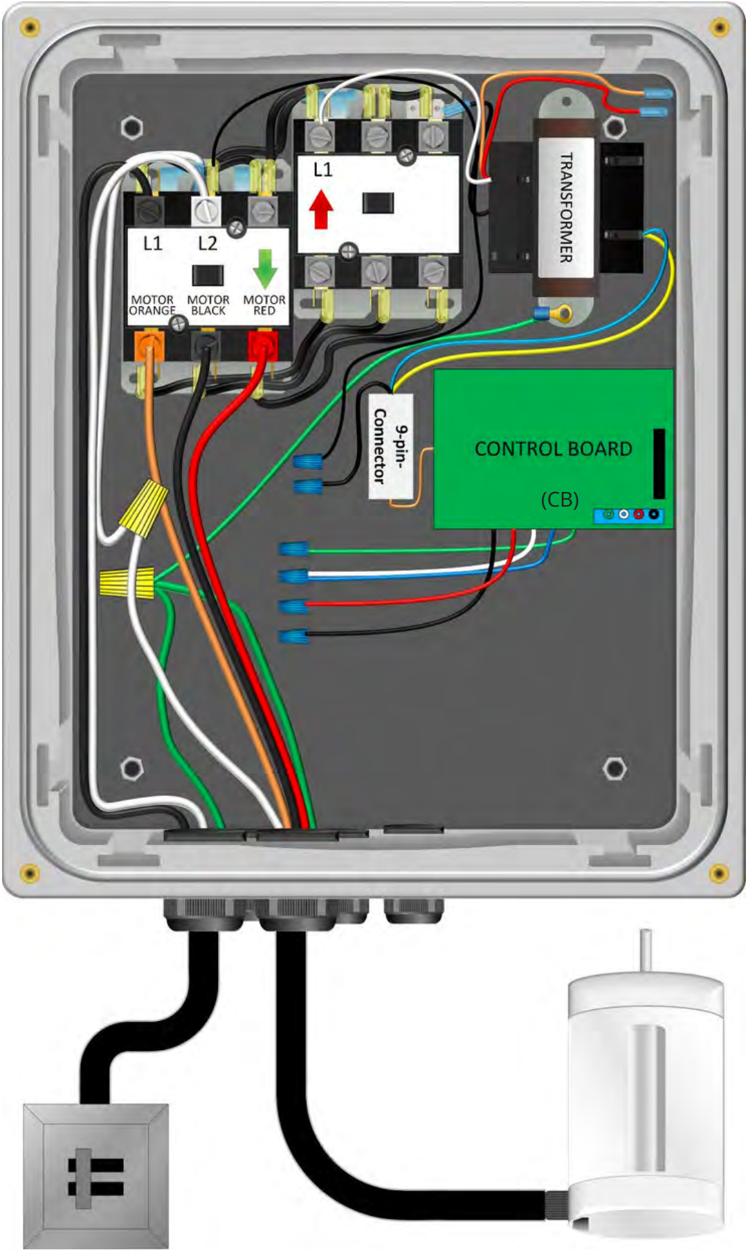
120 Volt Standard Lift Wiring
